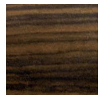
Dark Riverwood
